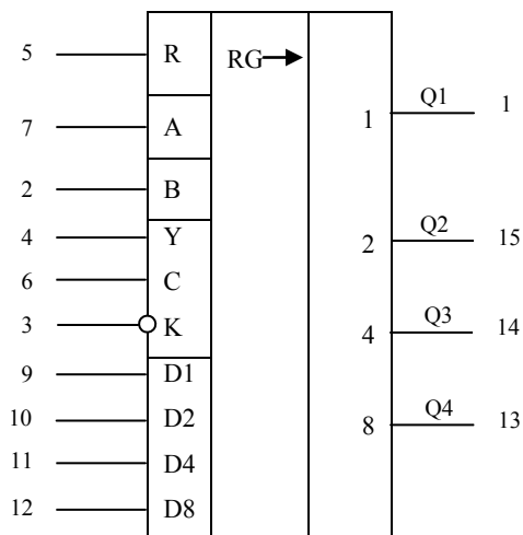
Условное графическое обозначение
